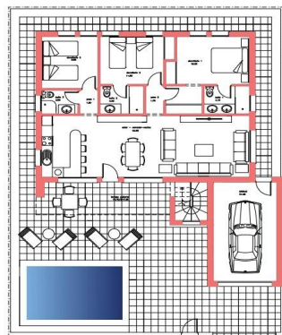
PLANTA BAJA
