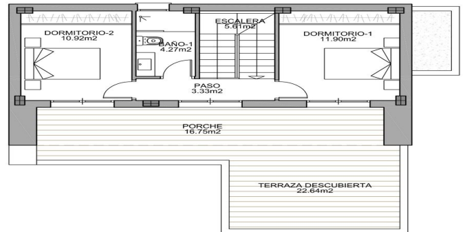
PLANTA PRIMERA
