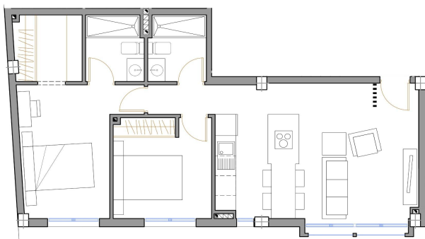
PLANTA PRIMERA, SEGUNDA Y TERCERA
