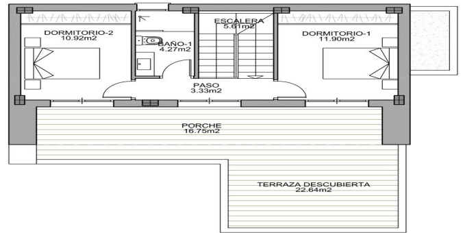
PLANTA PRIMERA
