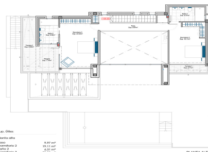
PLANTA ALTA
