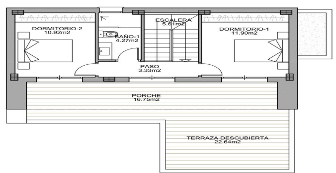
PLANTA PRIMERA
